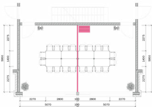
Grundrisse mit mobiler Trennwand
